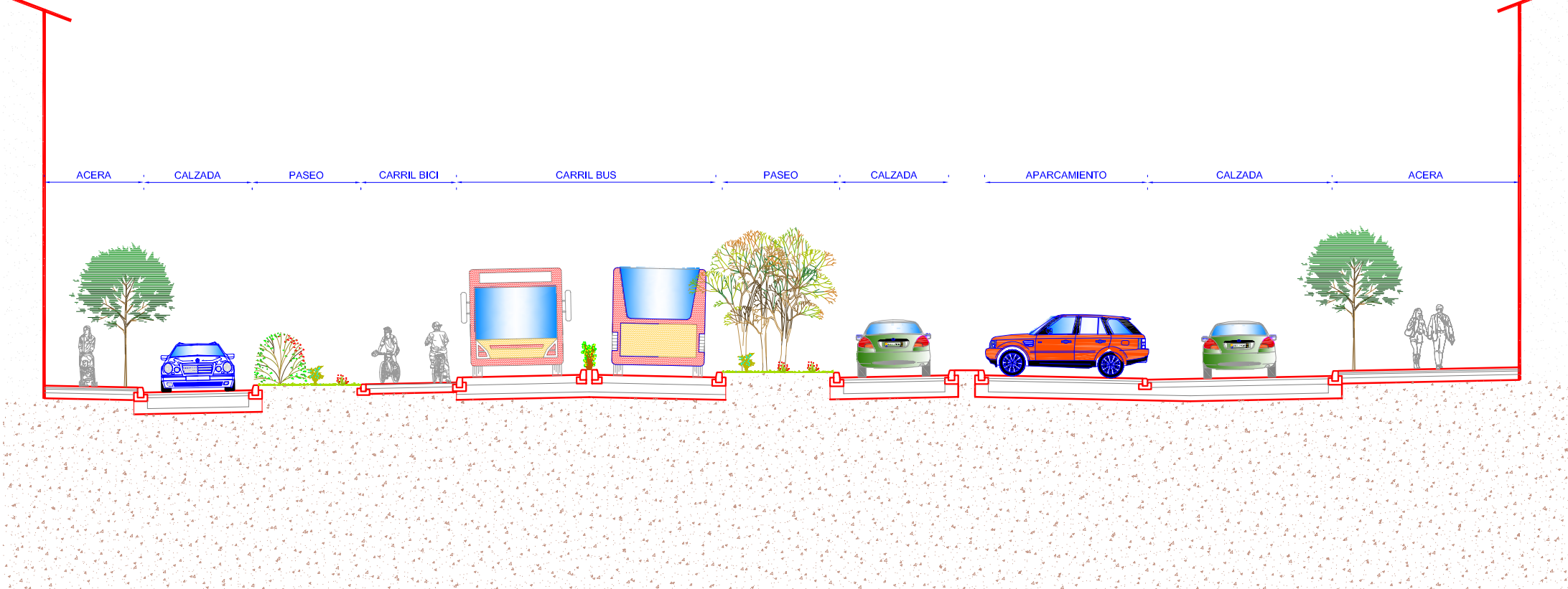
SECCION TIPO (LLEGADA A C/ SAENZ DE ALVARADO) E.: 1/150
