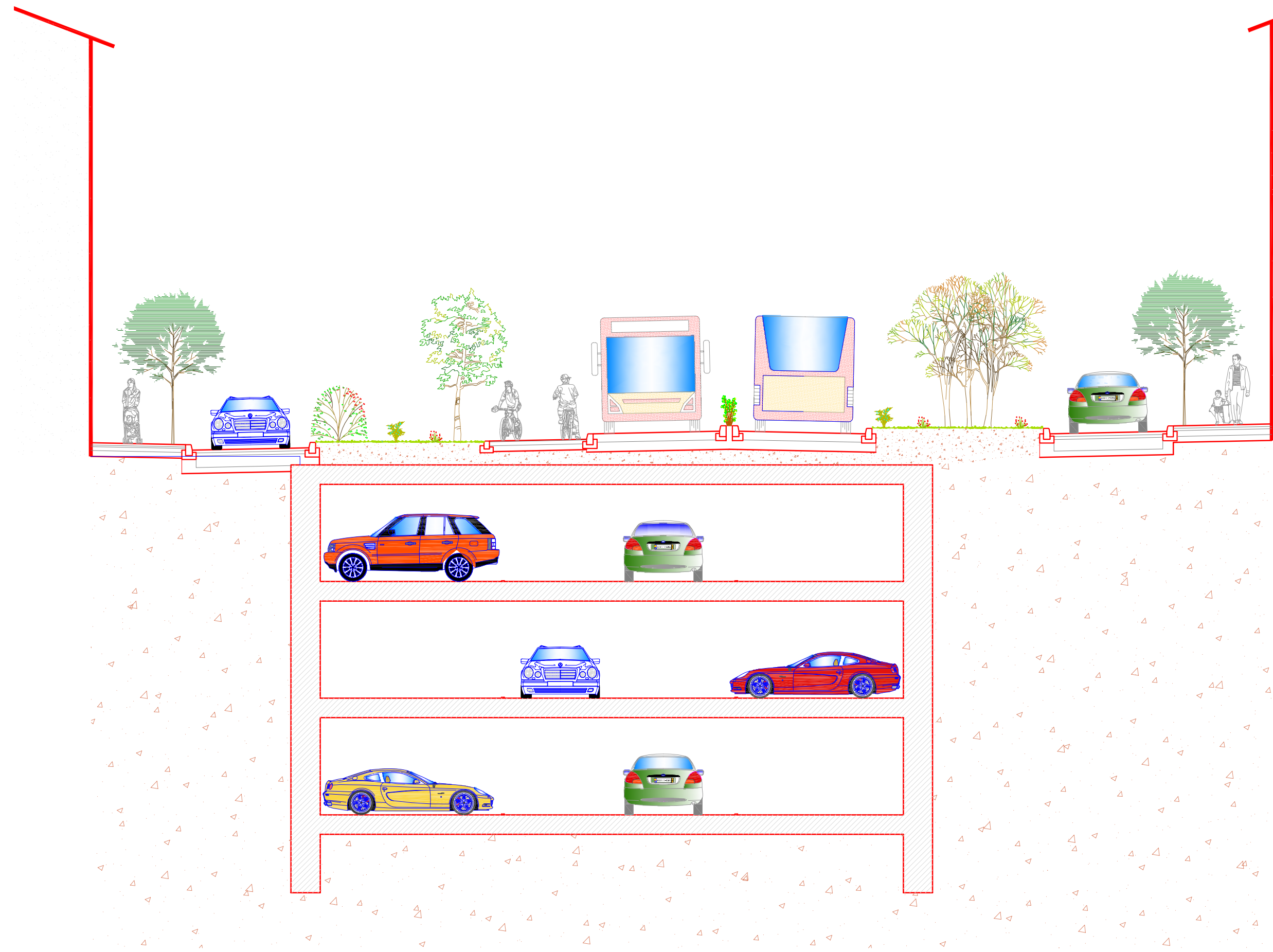
SECCION A-A1 E.: 1/100
