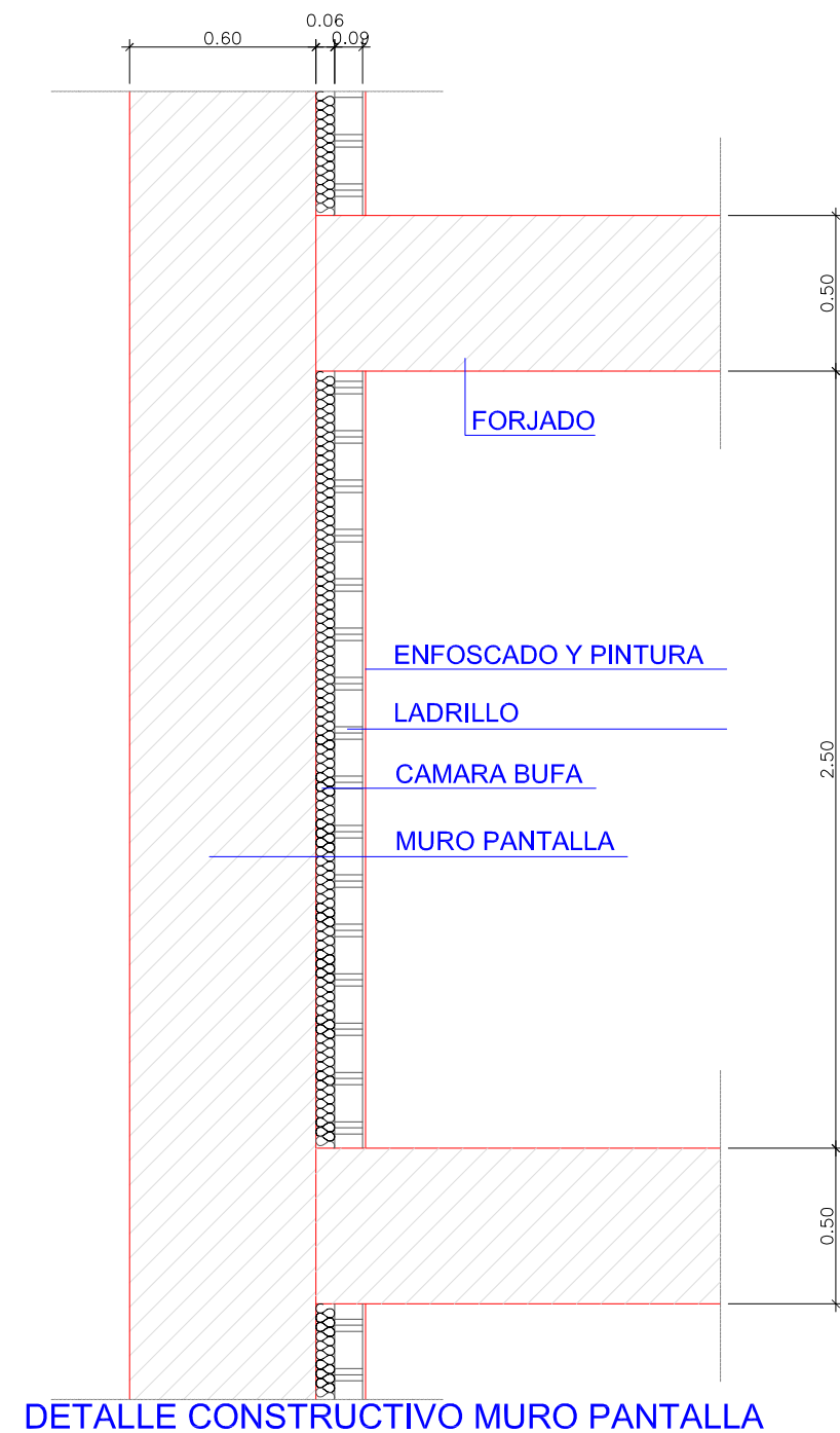
DETALLE CONSTRUCTIVO MURO PANTALLA
