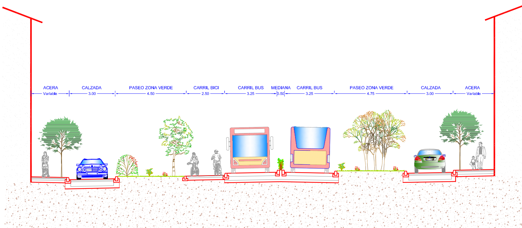
SECCION TIPO (ENTRE C/ SANTIAGO Y RUIZ PICASSO) E.: 1/150
