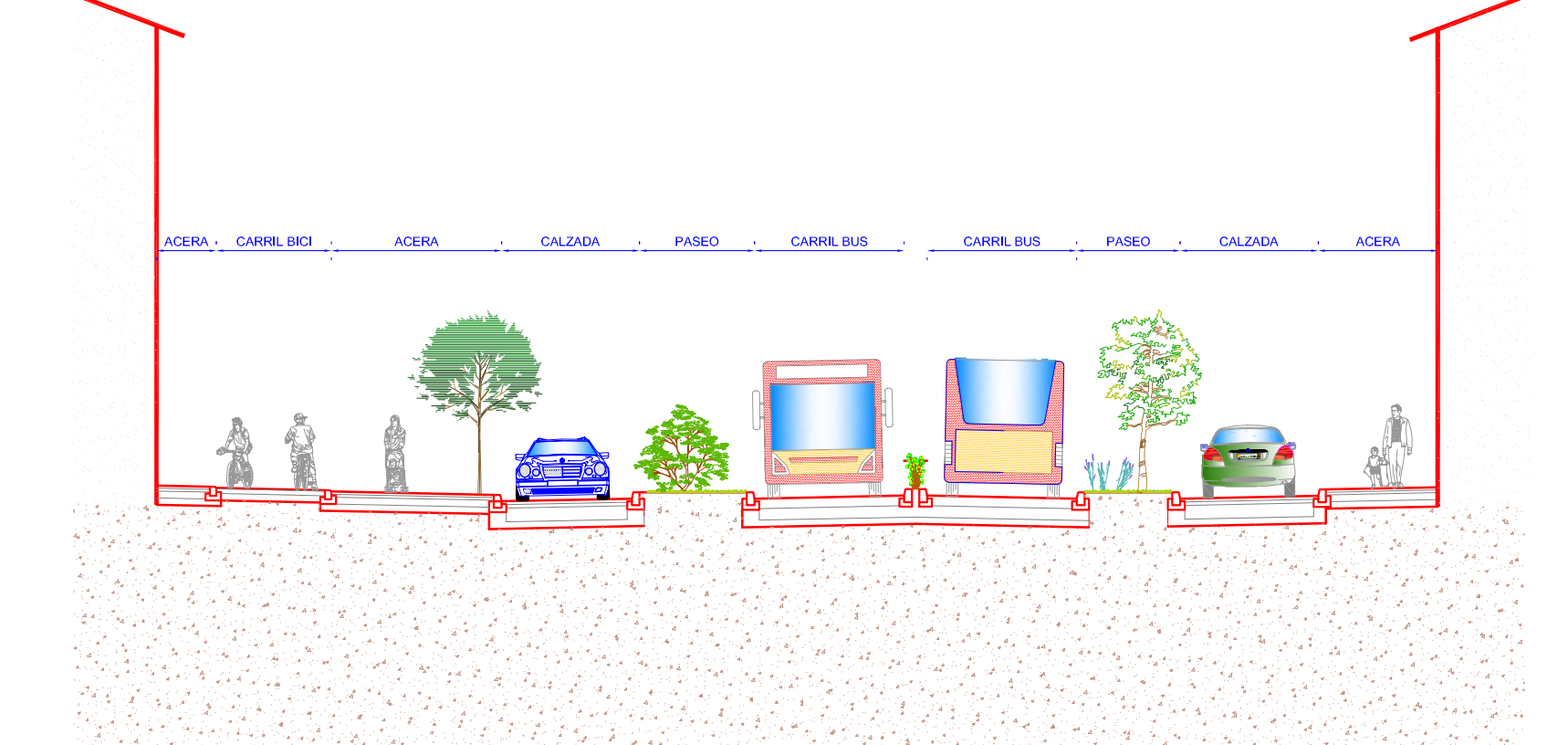
SECCION TIPO (FRENTE A SANTA Mª LA REAL ANTIGUA) E.: 1/150
